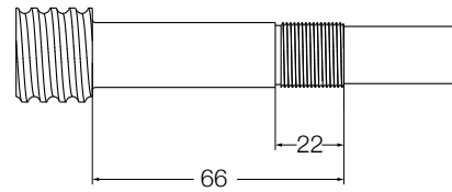
Endenbearbeitung Typ 4A für PND 25 x 5
